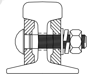
레일 정면도
