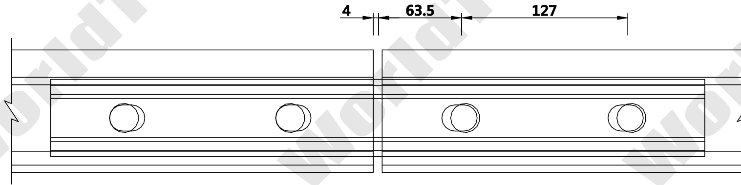
레일 측면도
