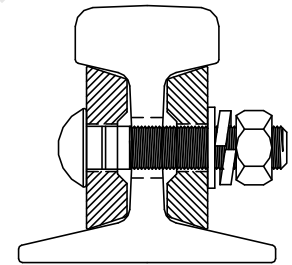
레일 정면도
