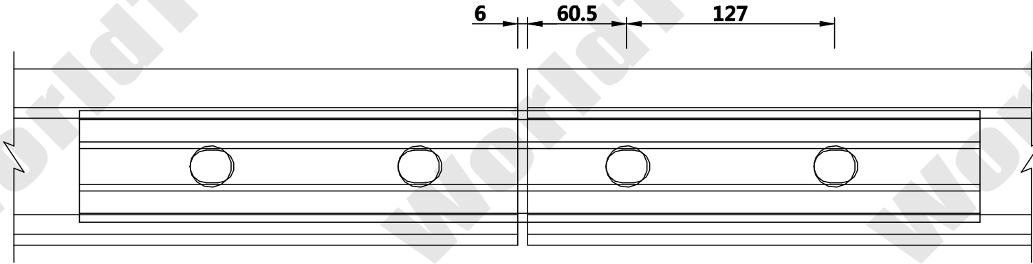
레일 측면도
