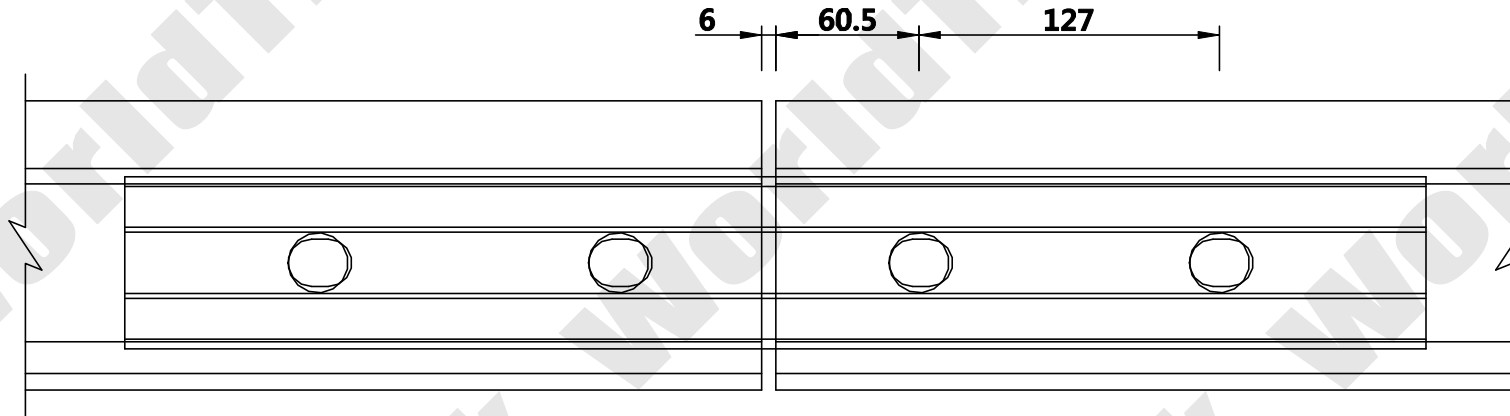
레일 측면도
