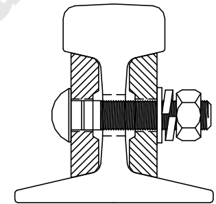
레일 정면도
