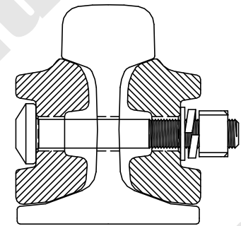
레일 정면도
