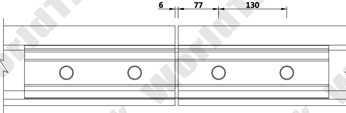
레일 측면도
