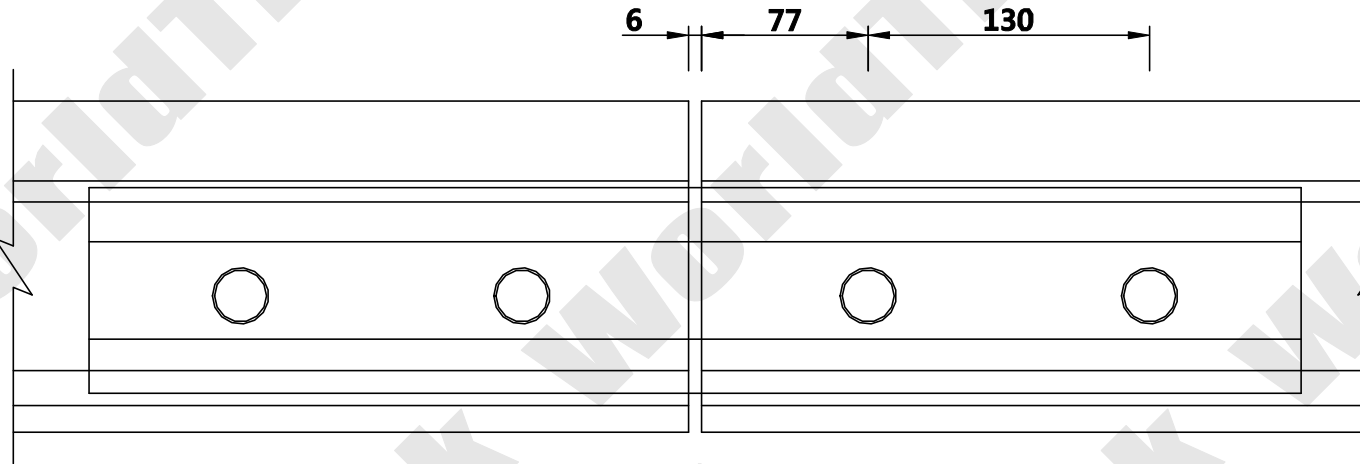
레일 측면도
