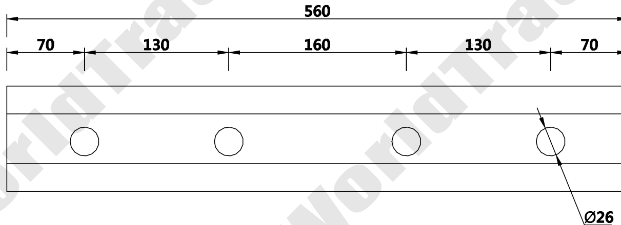
레일 측면도
