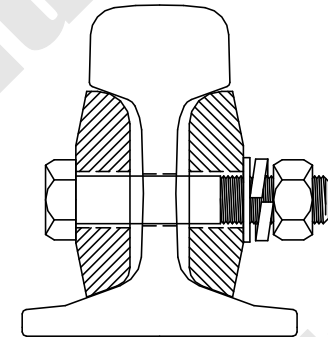
레일 정면도
