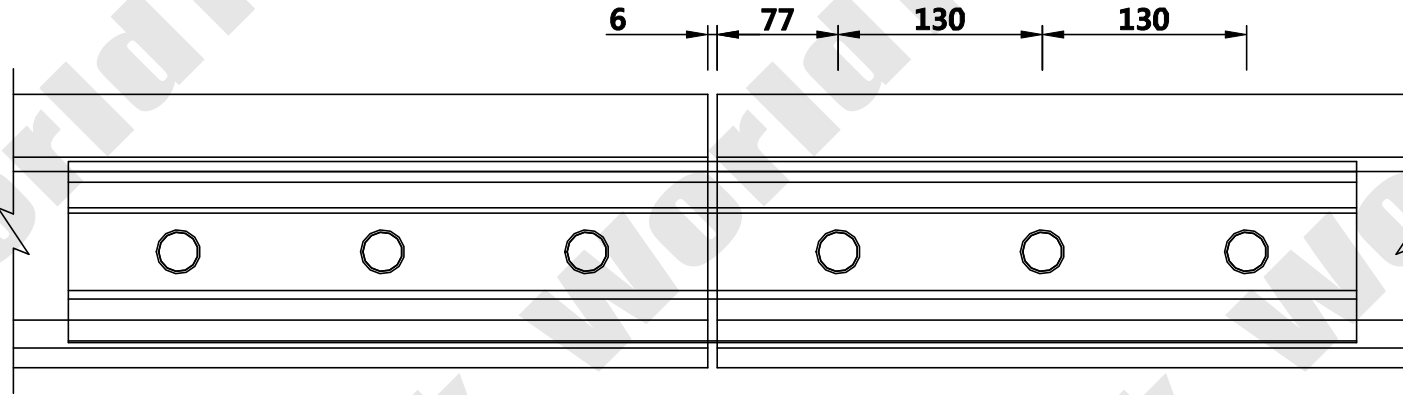
레일 측면도
