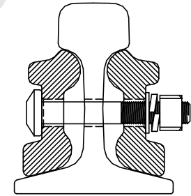
레일 정면도
