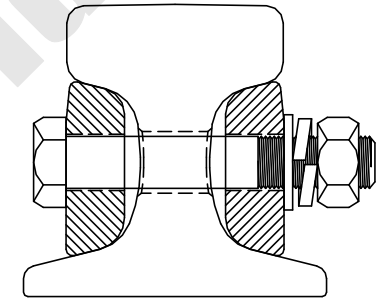
레일 정면도
