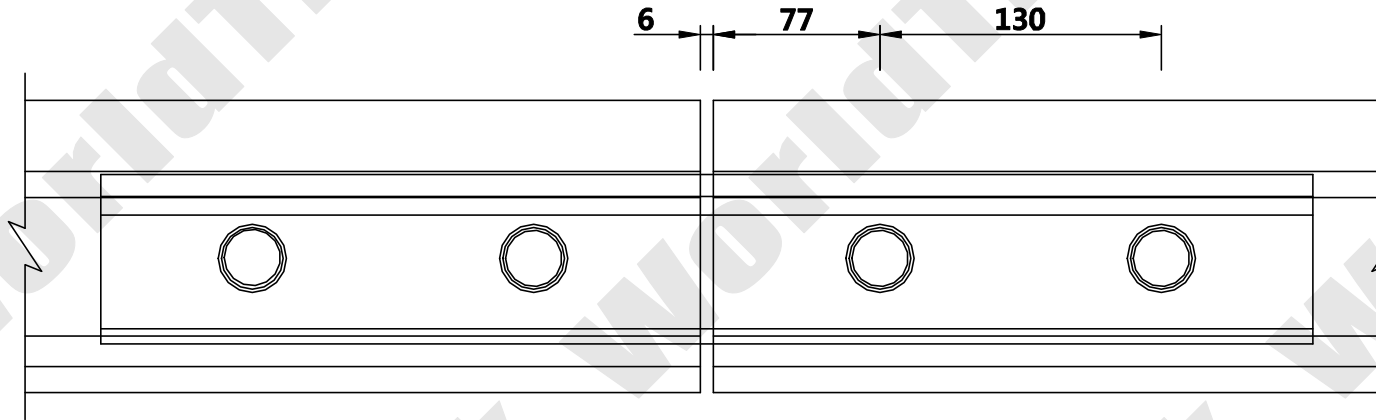
레일 측면도
